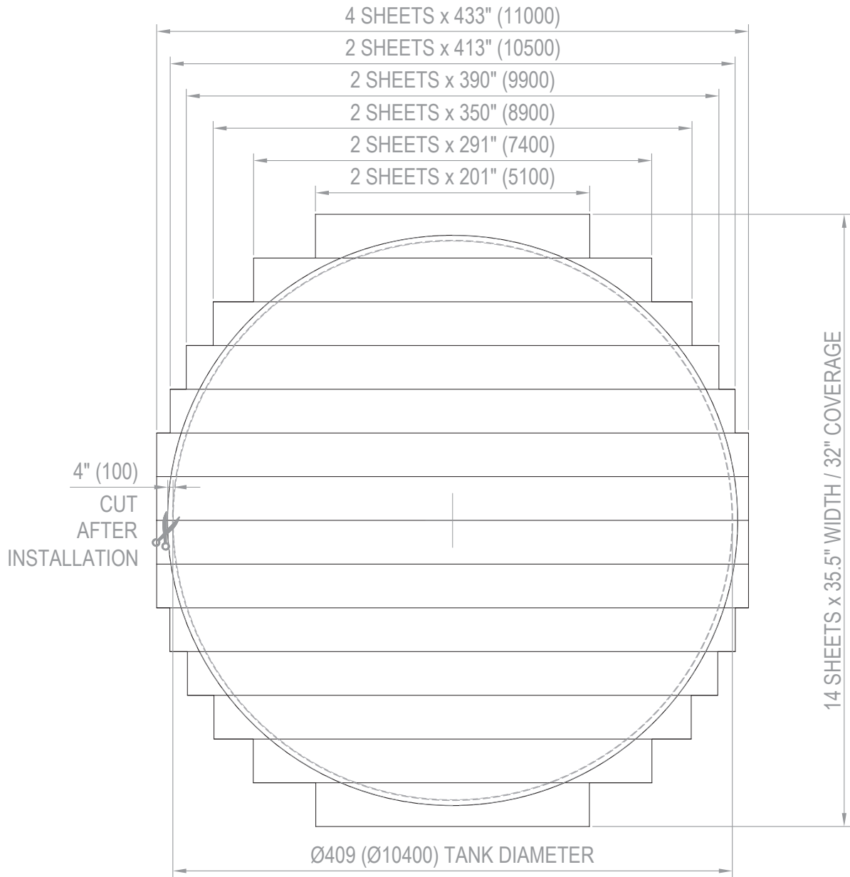
TANK PLAN SCALE: 1:100
