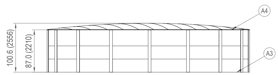
TANK ELEVATION SCALE: 1:100
