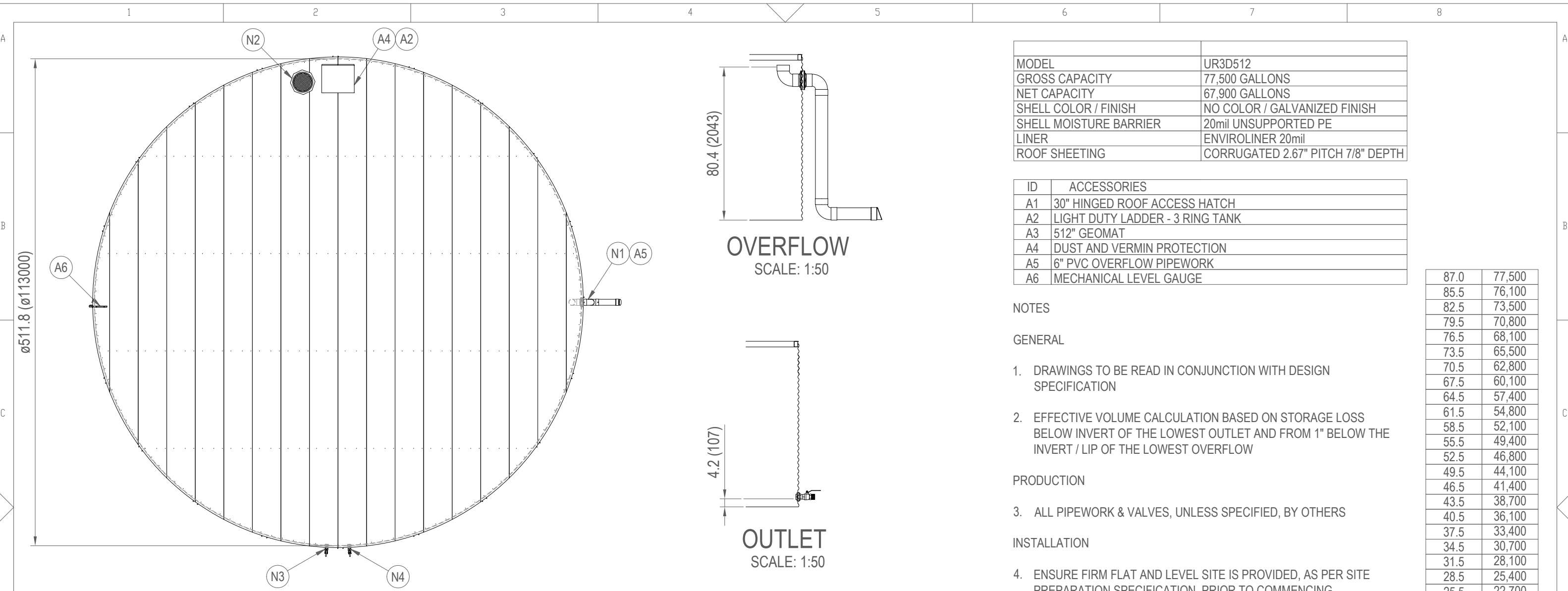
TANK PLAN SCALE: 1:100
